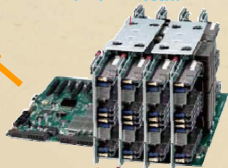
8Way 筐体内イメージ (5U/EIA規格)
